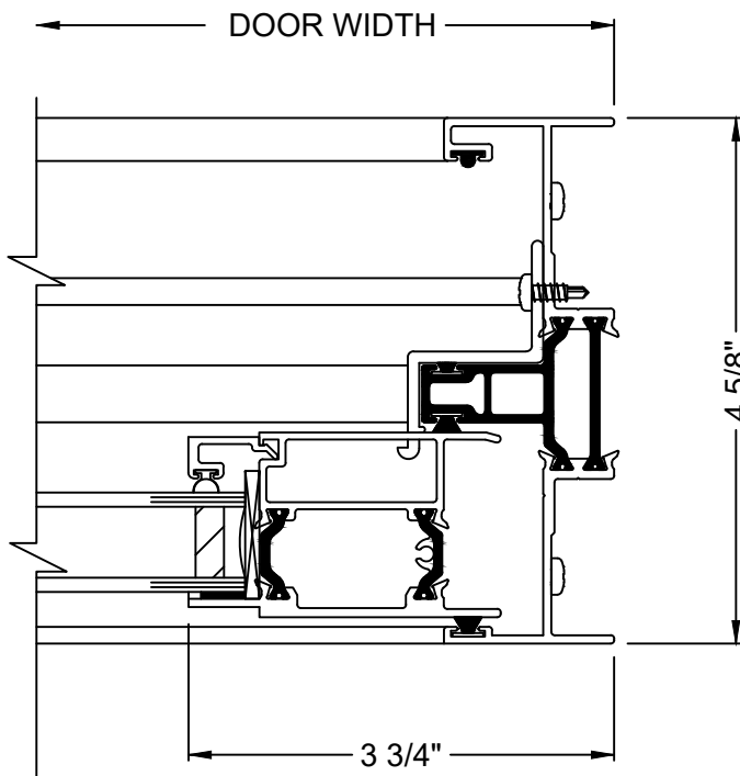
⑦ FIXED RIGHT JAMB
